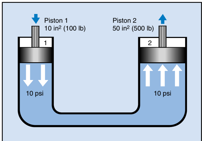
Fig. 1-8. Unequal piston areas
